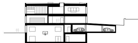
coupe transversale sur bâtiment B
